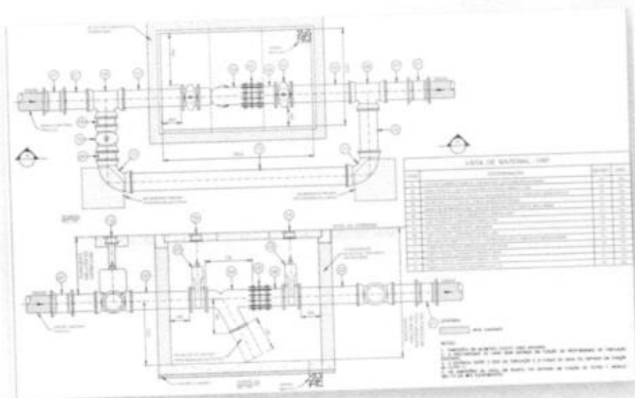
Projeto do filtro de linha que está sendo instalado na adutora proveniente do sistema produtor do Itatinga
